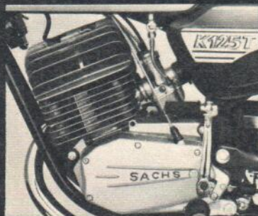
Sachs-Motor mit Superbreitwandzylinder. 17 PS, 6-Gang-Getriebe, 120 km/h.
