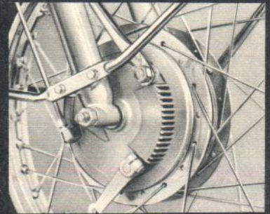
Große Alu-Vollnaben-Bremse. 160 mm Ø.
