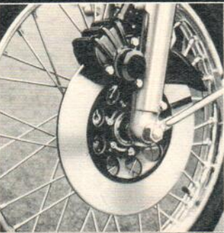
Neue Gabel mit langem Federweg Großdimensionierte mechanische Scheibenbremse
